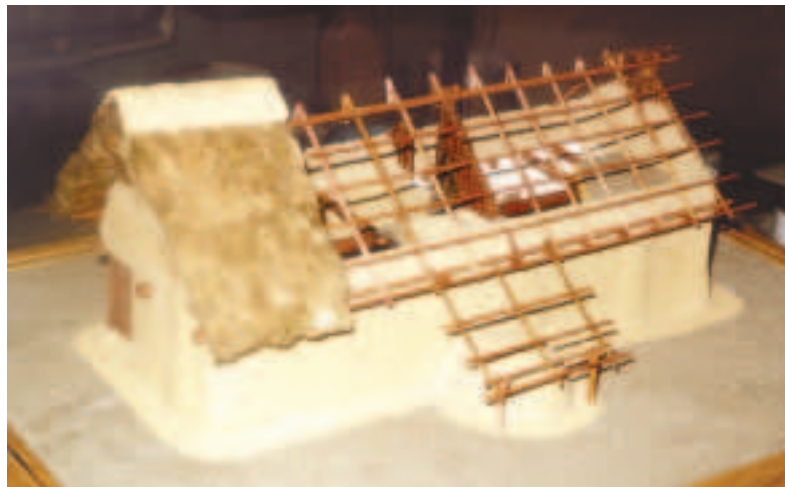
59. 15. századi kun ház rekonstrukciós modellje. Szentkirály
