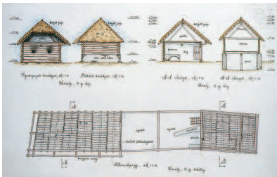
51. Késő középkori lakóház rekonstrukciója Sarvalyról
