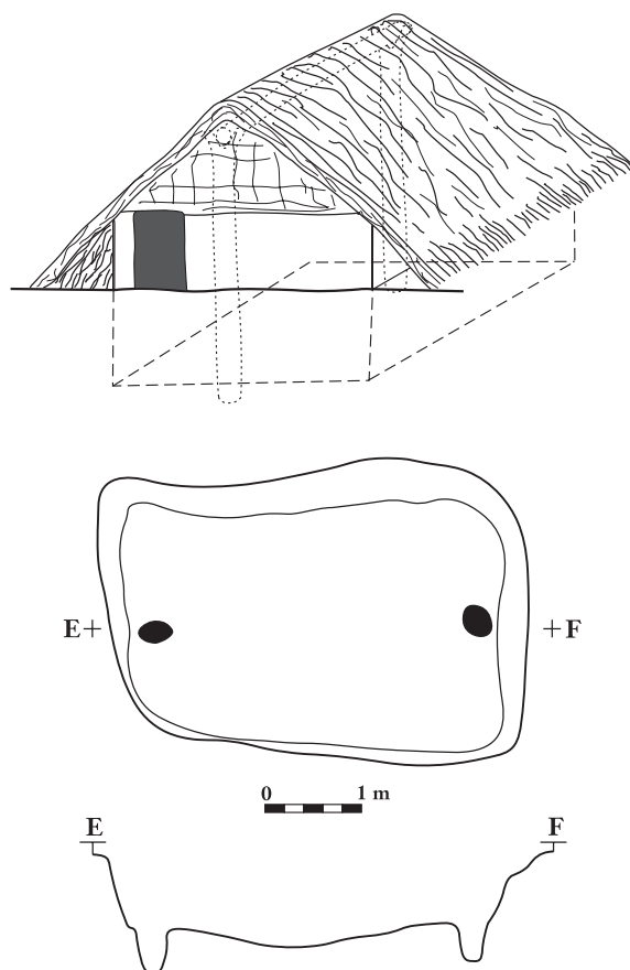
45. Földbe mélyített gödörlakás alaprajza és rekonstrukciója. Ménfőcsanak–Bevásárlóközpont, 225. objektum
