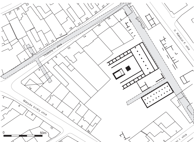
20. Savaria délnyugati városrésze az Isis-szentéllyel
