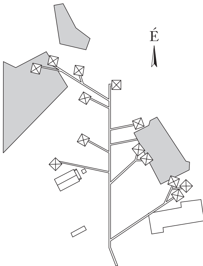
33. Aquincum. A vízvezeték kizsgáló kutak a Római-parton
