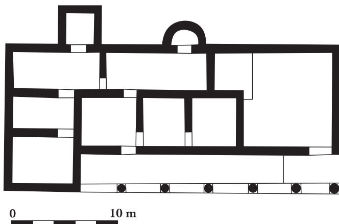
38. Porticus villa alaprajza. Csúcshegy
