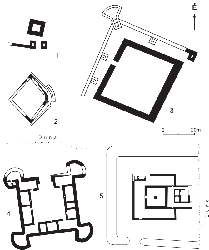
6. Késő római kiserődök: 1 – Lussonium (Dunakömlőd), 2 – Cirpi (Dunabogdány), 3 – Azaum (Almásfüzitő), 4 – Visegrád–Gízella telep, 5 – Solva-19 (Pilismarót–Malompatak)
