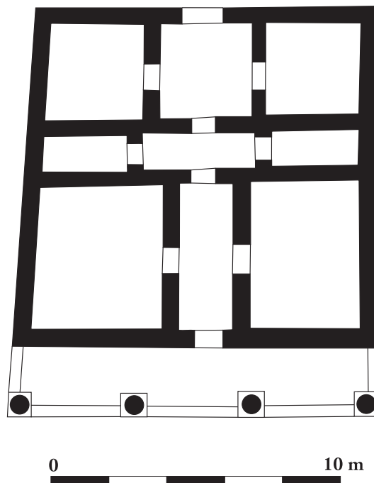
39. Középfolyosós villa. Békásmegyér, 3. sz. villa
