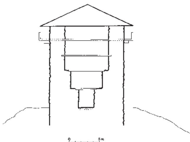
11. A ságvári őrtorony rekonstrukciós metszete
